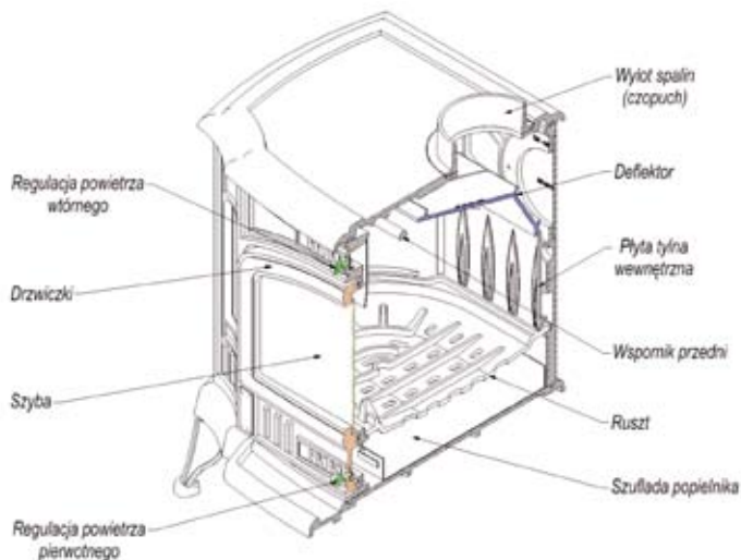
Rys. 1 Kozia K9- opis elementów
